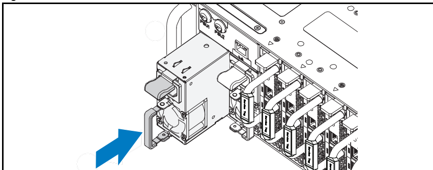
Figure 1-8. Installation d'un bloc d'alimentation
