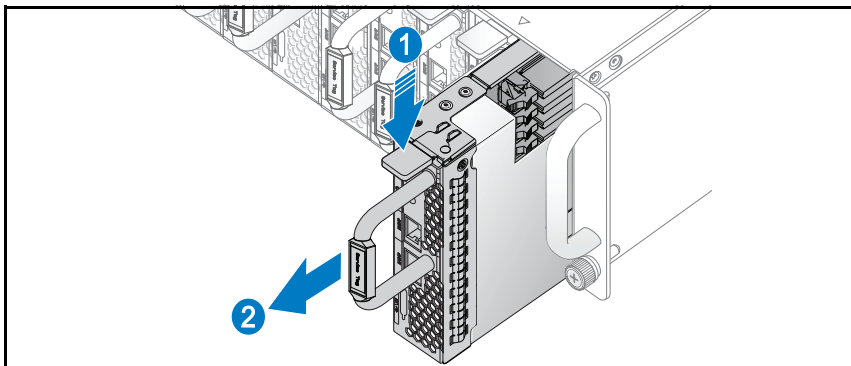
Рис. 1-6. Извлечение салазок
