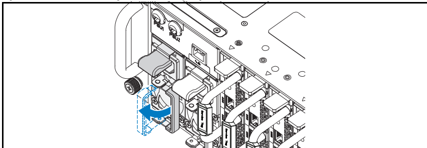
Rycina 1-4. Odblokowywanie uchwytu jednostki zasilacza
