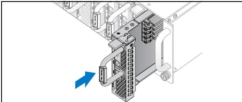
Рис. 1-12. Установка салазок
