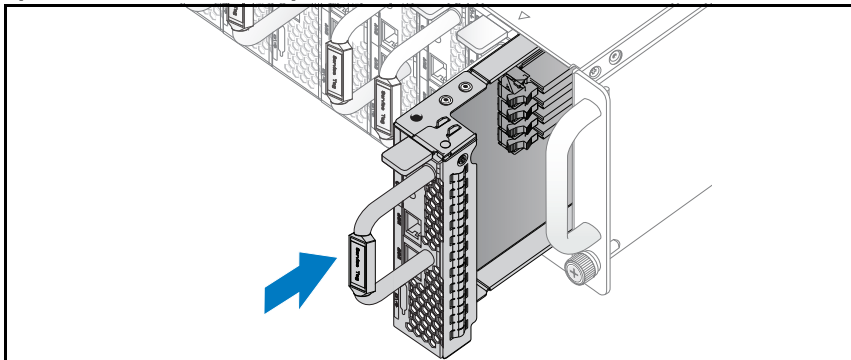
Rycina 1-12. Instalowanie dysków SLED
