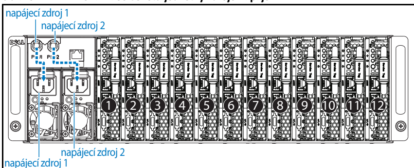
Obrázek 1-11. Lokalizace soketů jednotky zdroje napájení
